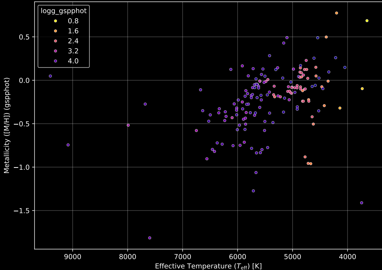
APOGEE DR17 Field: [284-31-O_TESS] Stellar Population Parameters (n= 163)
