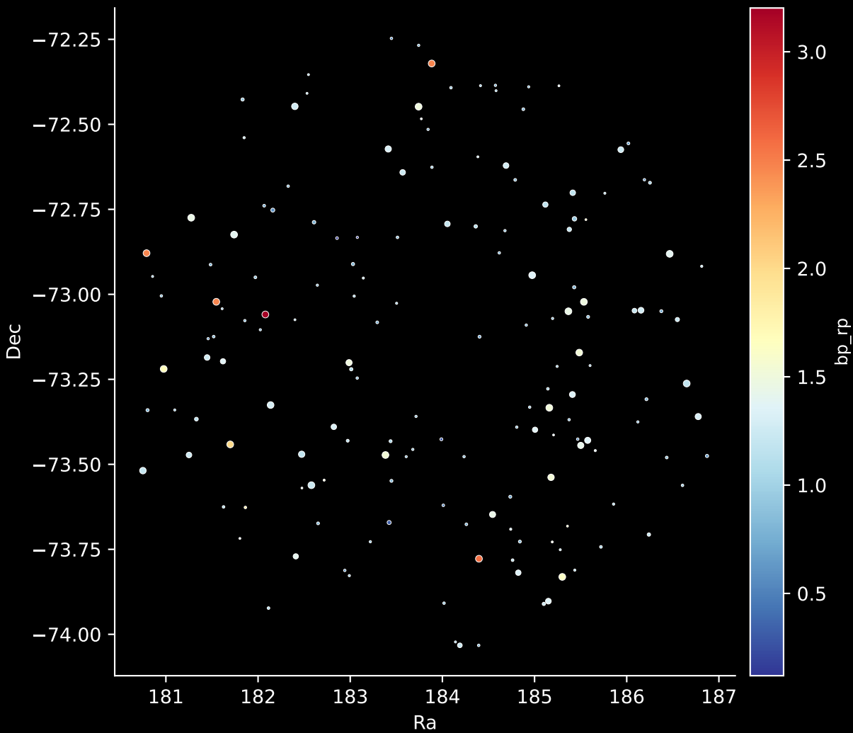
APOGEE DR17 Field: [284-31-O_TESS] Stars: 163
